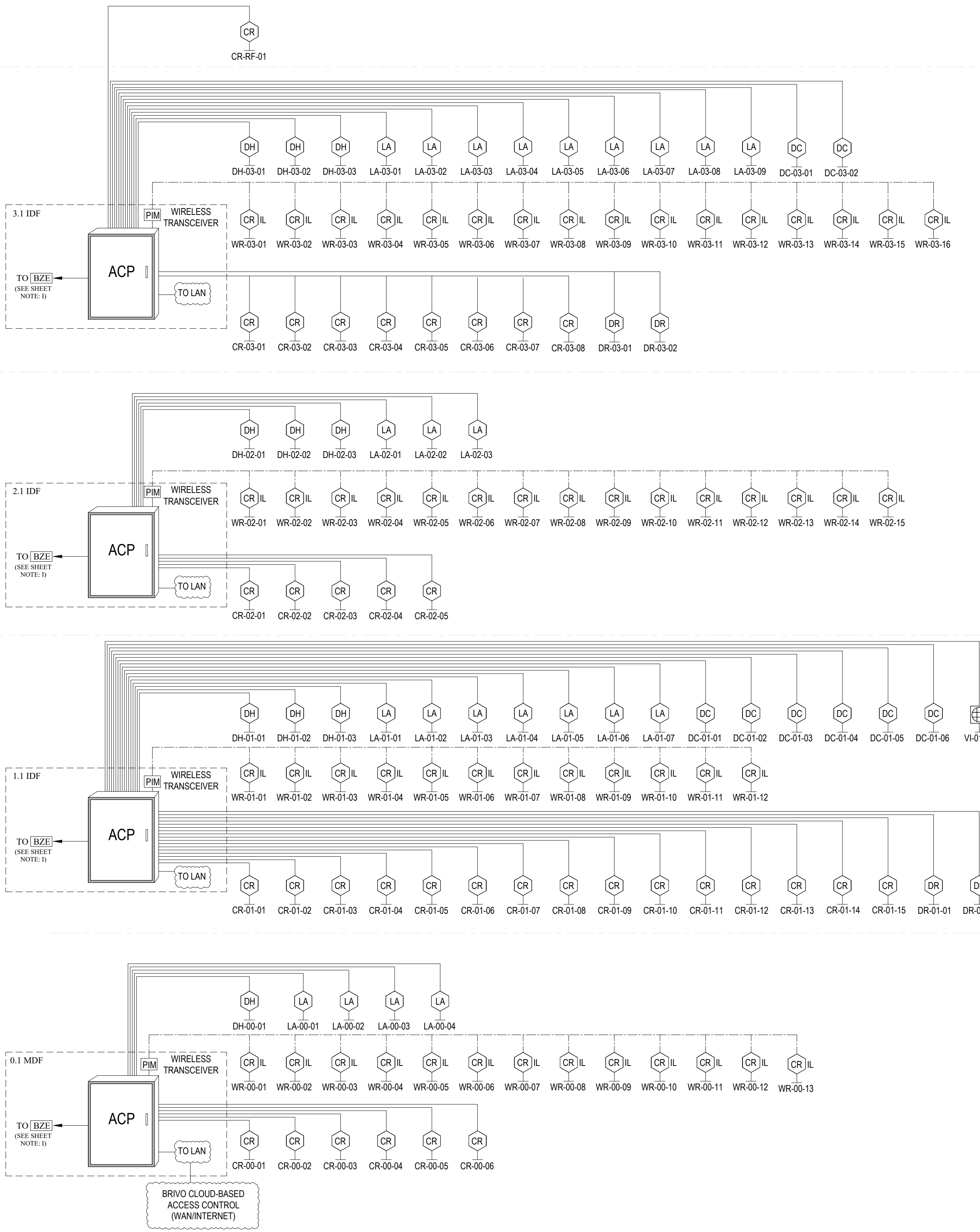
ACCESS CONTROL SYSTEM RISER DIAGRAM SCALE: N.T.S.
